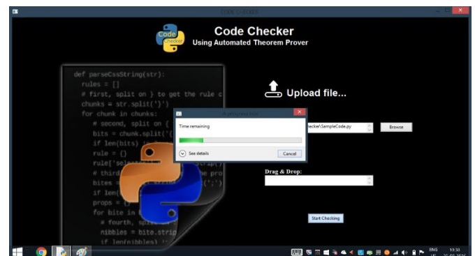
Fig. 5. Progress Bar
